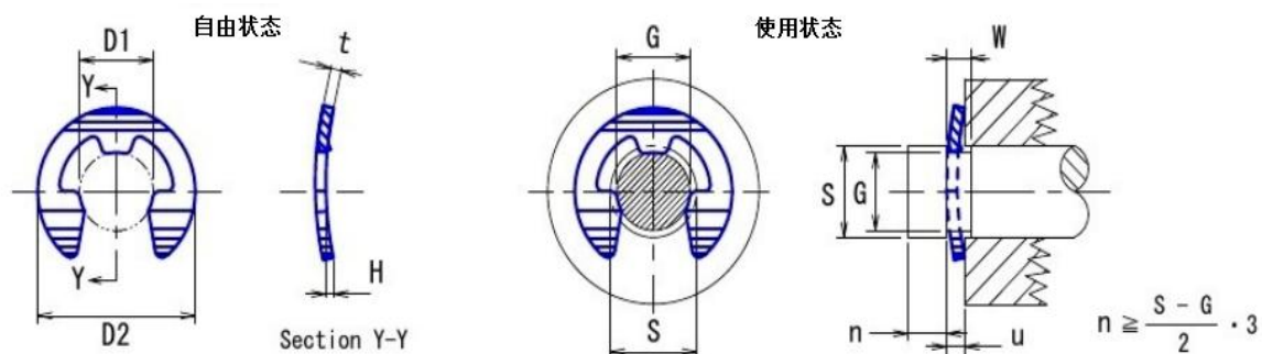
IWT 弯曲BE型挡圈规格表 (轴用)
